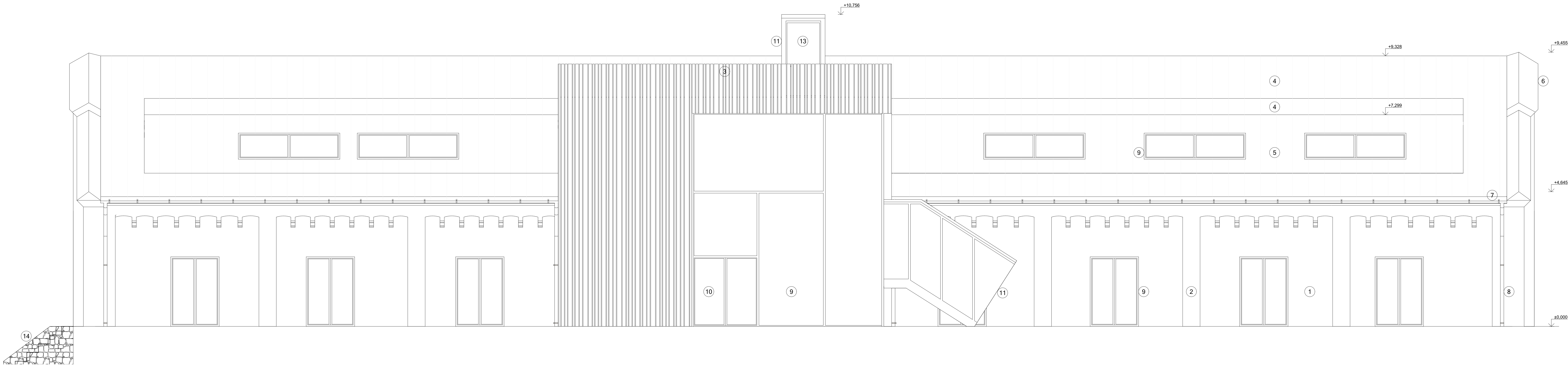
JIHOZÁPADNÍ POHLED
